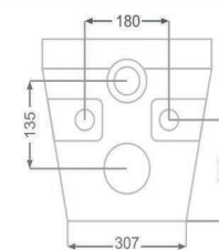
کاتیا ۵۶ (سیستم تخلیه آبشاری)
