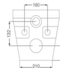
سانتا (سیستم تخلیه آبشاری - بدون ریم)
